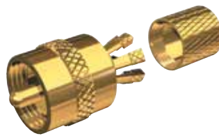
LODDEFRIT PL259 STIK Passer til RG58 og 8X kabel guldbelagt.
